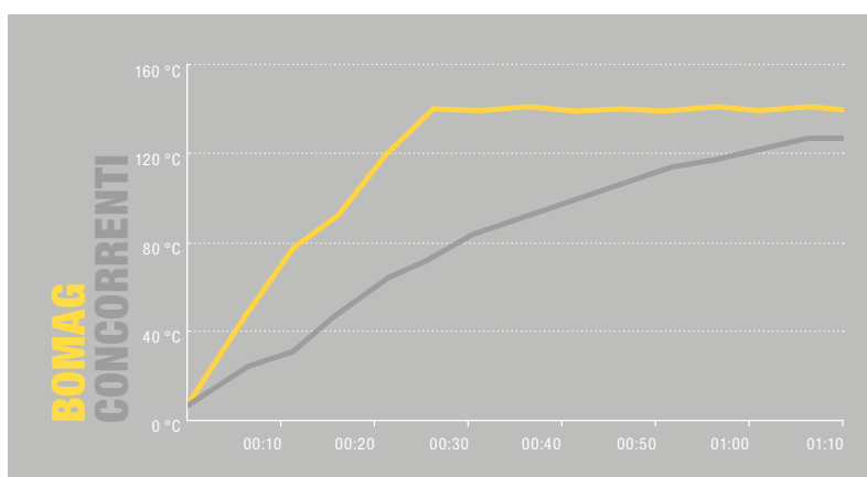
BOMAG rispetto ai banchi elettrici tradizionali: riscaldamento più veloce del 50 %.
